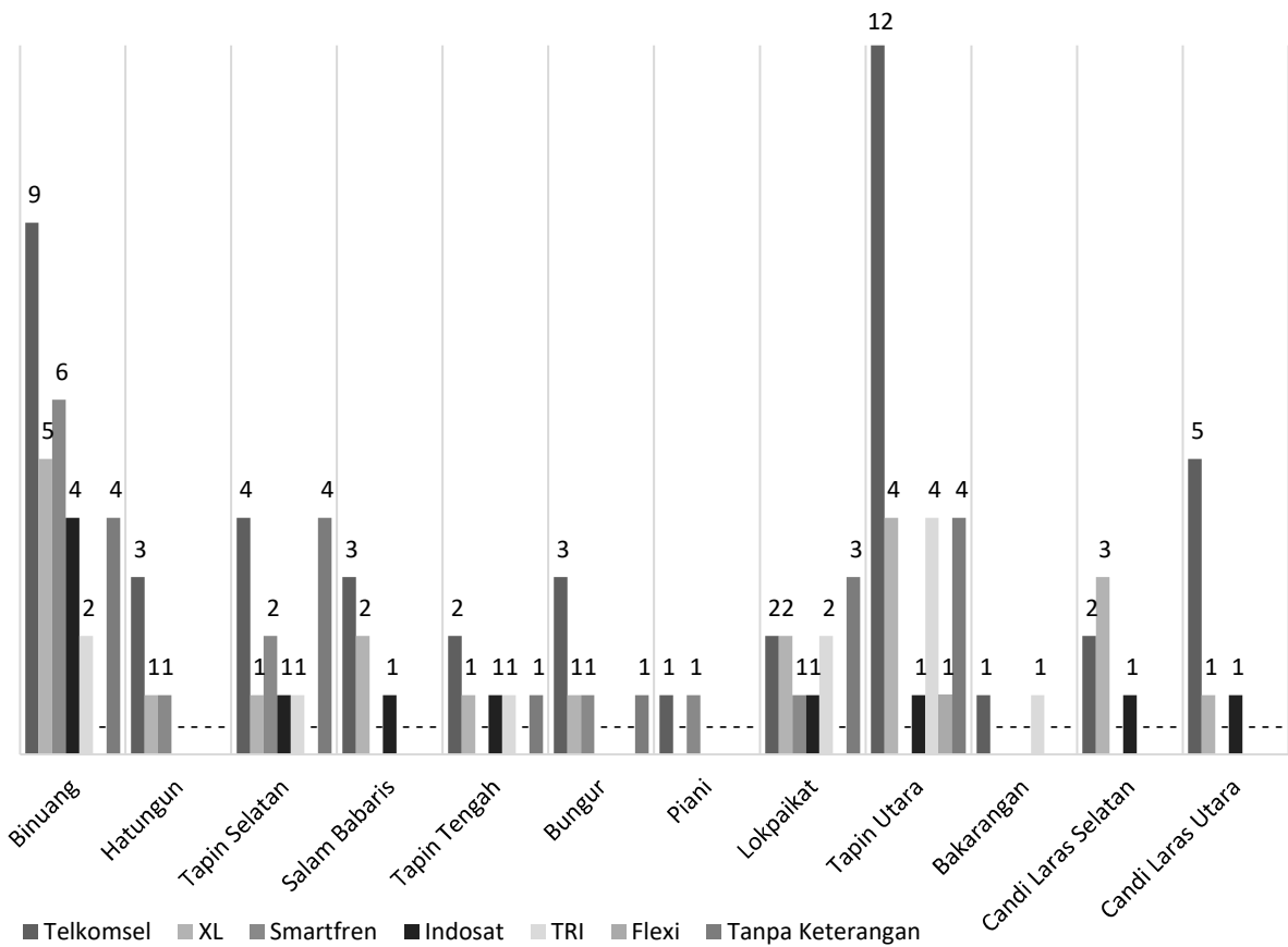
Diagram 12.4.4.1 Jumlah Menara BTS Swasta berdasarkan Operator per Kecamatan di Kabupaten Tapin Tahun 2022.
