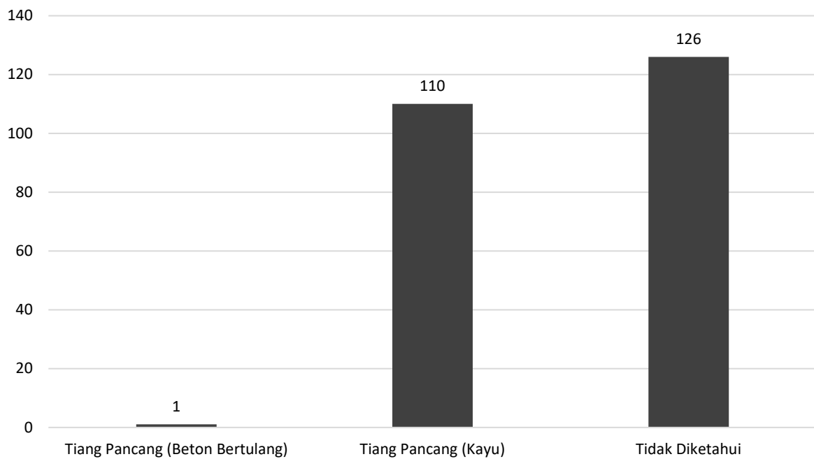
Diagram 25.11 Jumlah Jembatan berdasarkan Tipe Fondasi di Kabupaten Tapin Tahun 2022.
