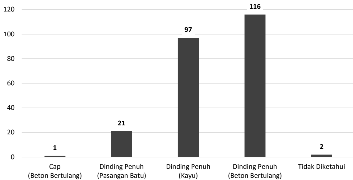
Diagram 25.10 Jumlah Jembatan berdasarkan Tipe Bangunan Bawah di Kabupaten Tapin Tahun 2022.
